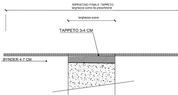
SEZIONE TIPOLOGICA Ripristino dello stato finale
