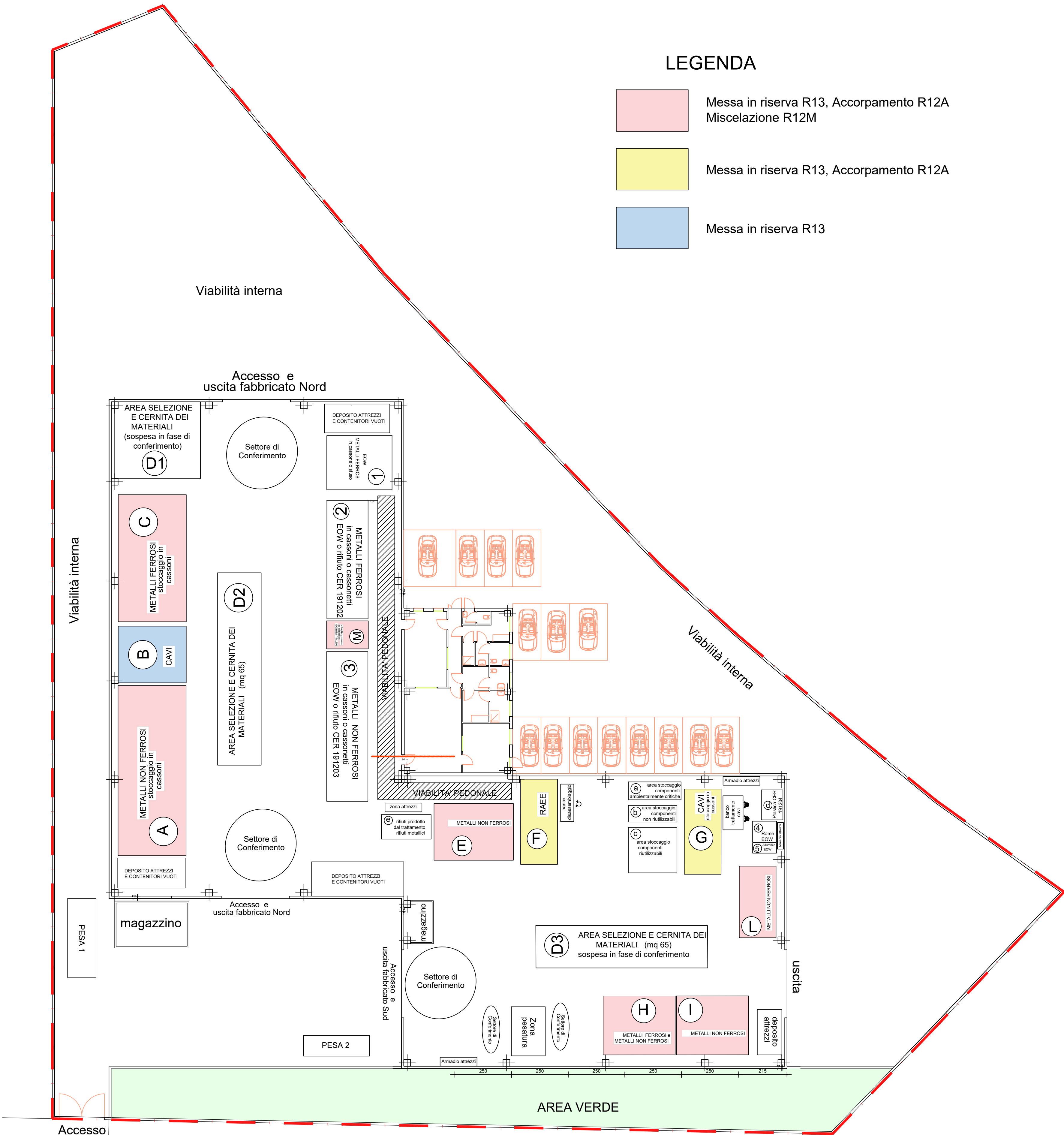
PLANIMETRIA GENERALE scala 1:250
