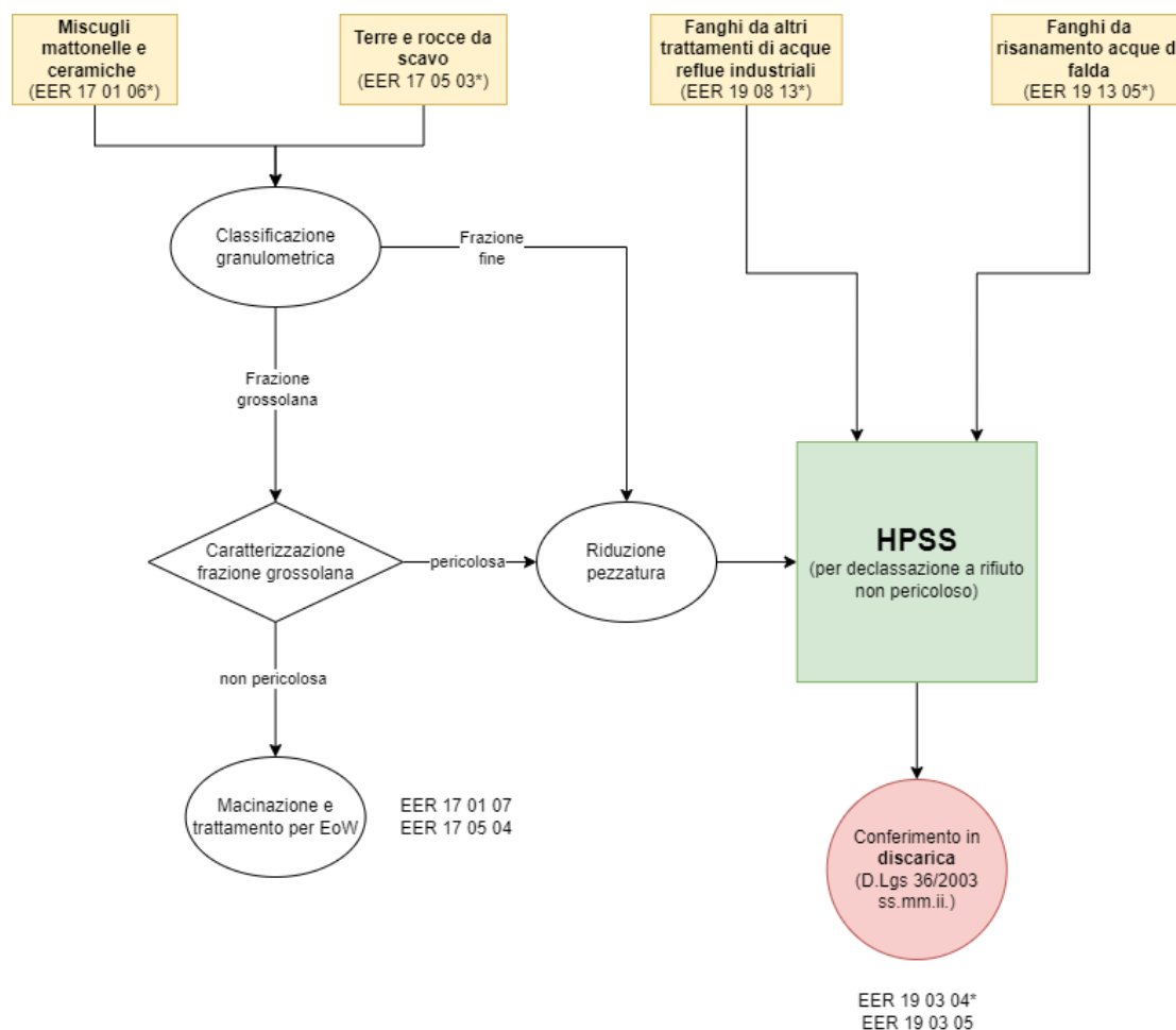
Figura 4.b: schema di trattamento di rifiuti in ingresso classificati come pericolosi
