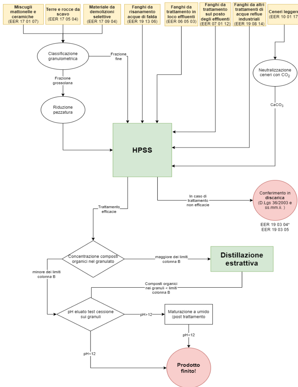
Figura 4.a: diagramma di flusso dei vari rifiuti non pericolosi trattabili dall'impianto nelle varie sezioni impiantistiche
