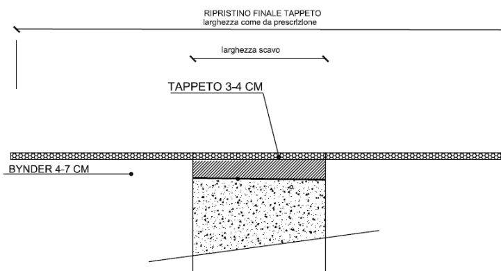
SEZIONE TIPOLOGICA Ripristino dello stato finale
