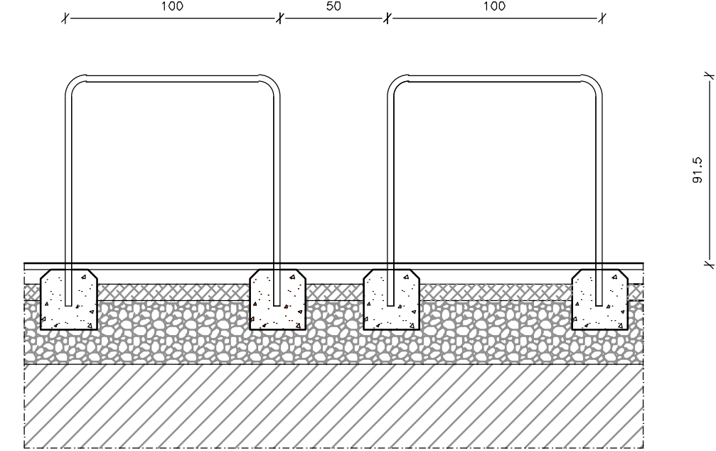
DISSUASORE TIPO
