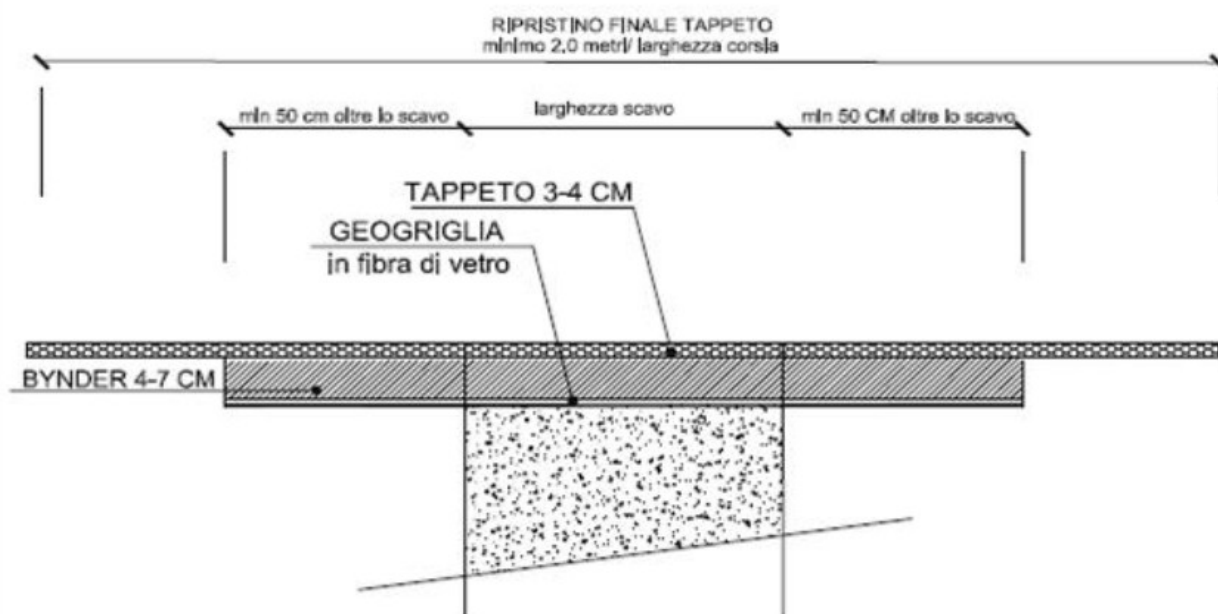
SEZIONE TIPOLOGICA Ripristino dello stato finale
