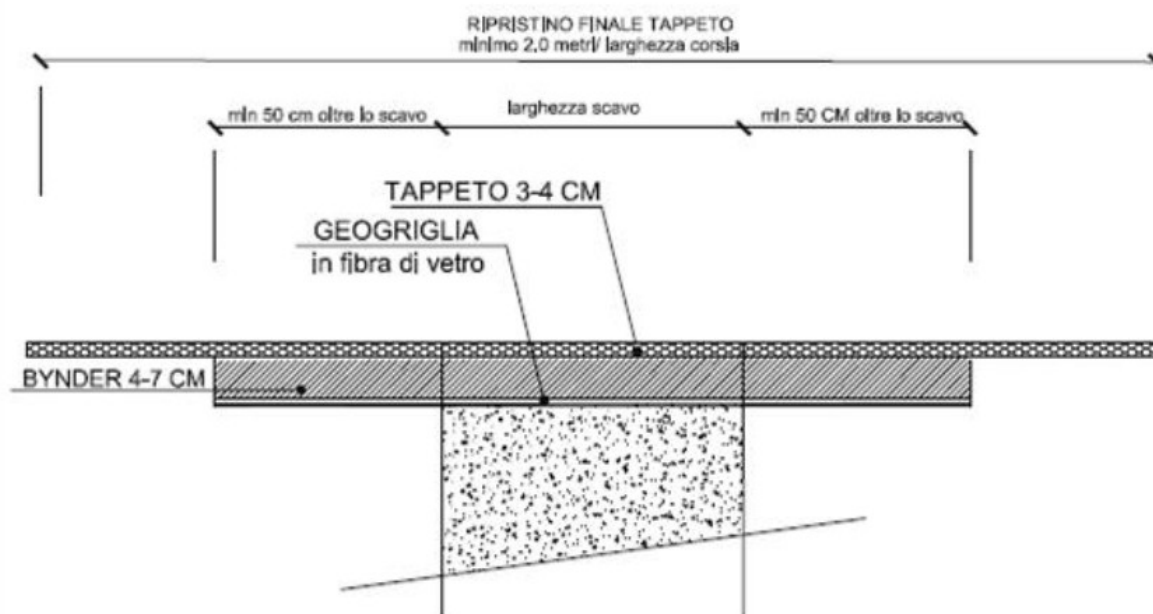
SEZIONE TIPOLOGICA Ripristino dello stato finale
